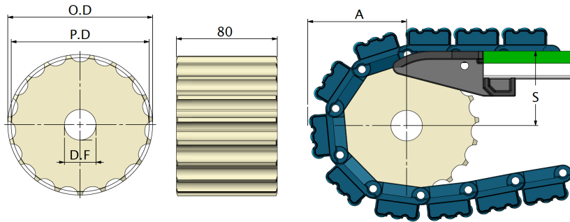
惰輪型號尺寸對照表
