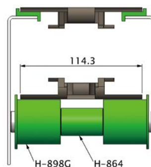
K450雙排
