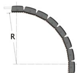
內徑最小轉彎半徑 R=300mm
