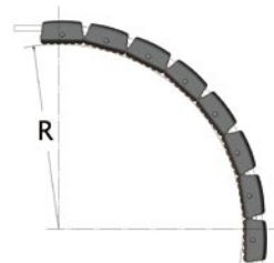
內徑最小轉彎半徑 R=500mm
