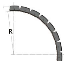
內徑最小轉彎半徑 R=400mm
