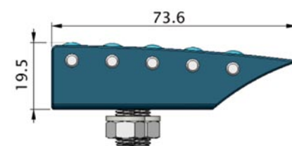
5列滾珠
