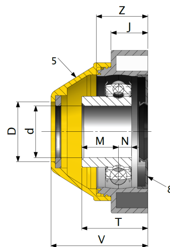
開孔式
