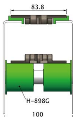
K330單排
