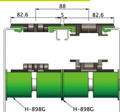
K325雙排
