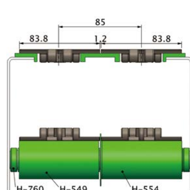
K330雙排
