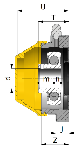
密閉式
